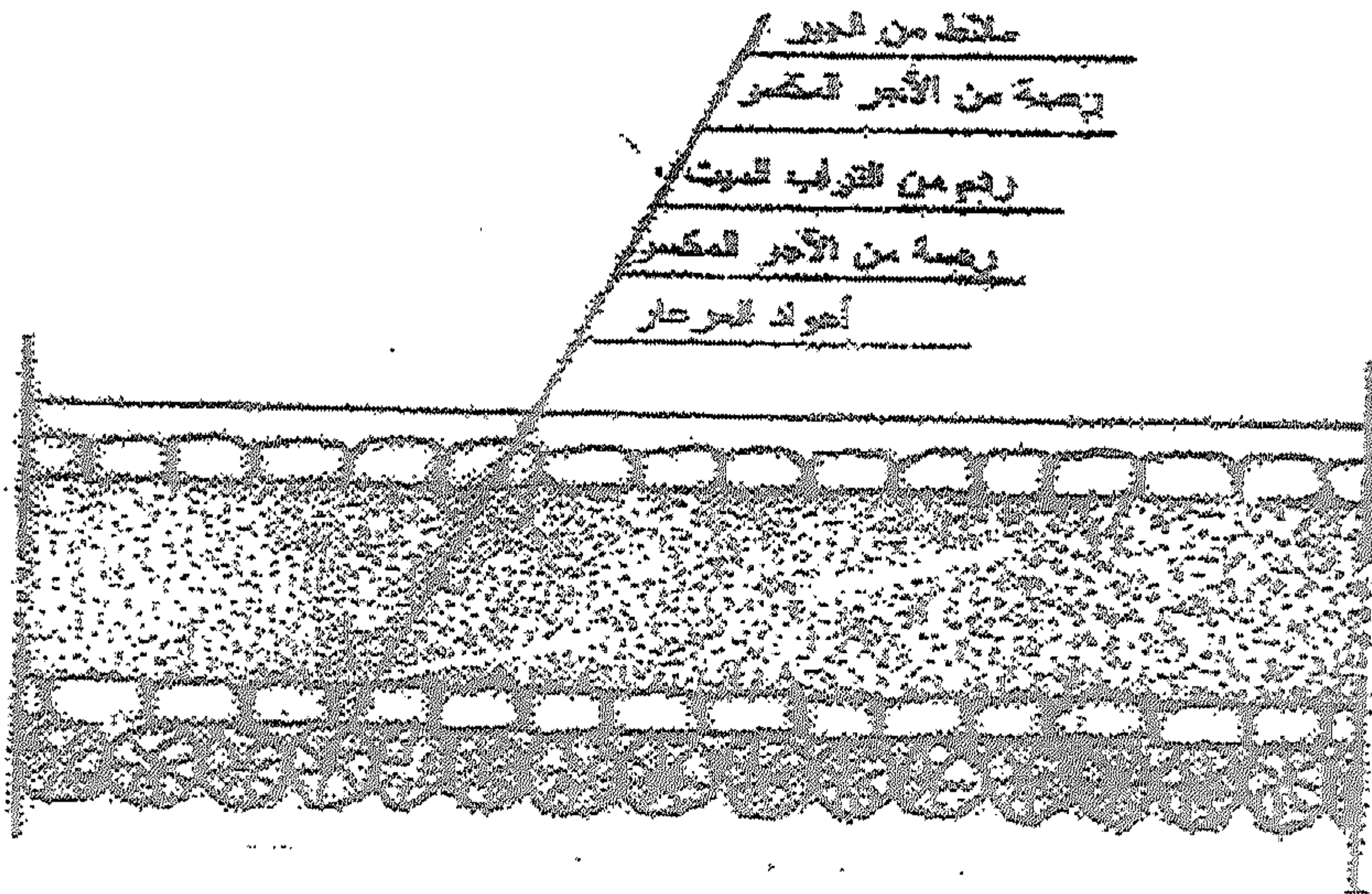
(شكل رقم ٨٤) مخطط نسقف من أعواد العرعر عن د/ نجوى عثمان.
